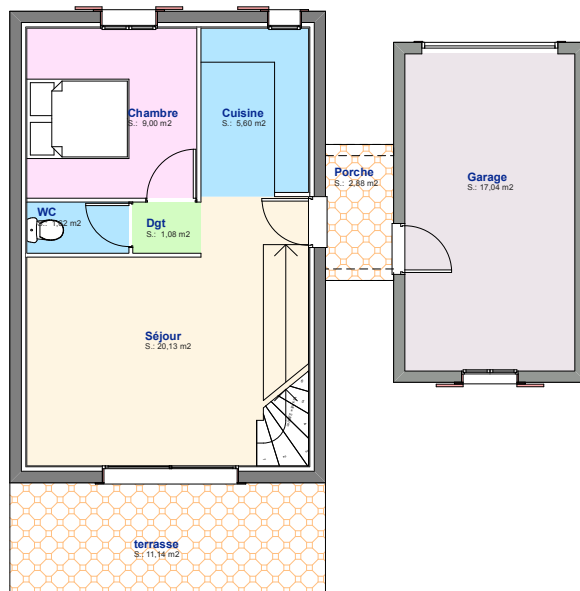
PLAN DE REZ CHAUSSEE
